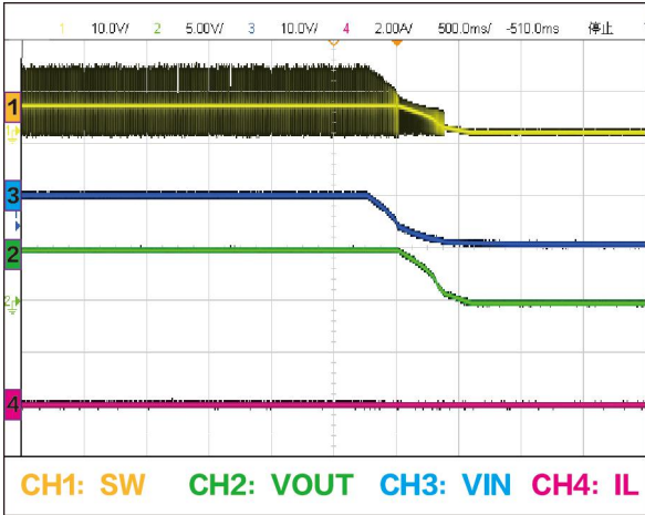
V_{IN}=12V V_{OUT}=5V 关闭波形 I_{OUT}=0A
