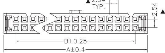
14P-64P 双槽
