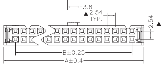
14P-64P 双槽
