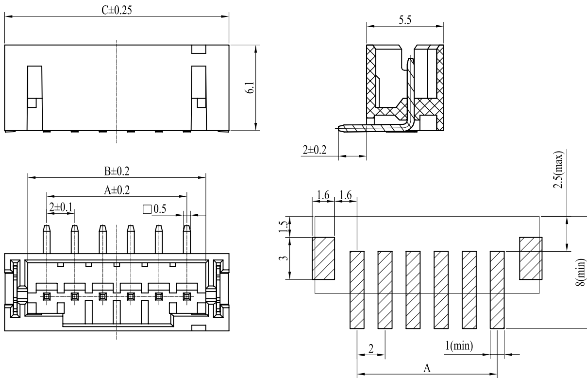
PCB板安装尺寸
