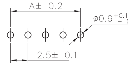
P.C.B LATOUT
