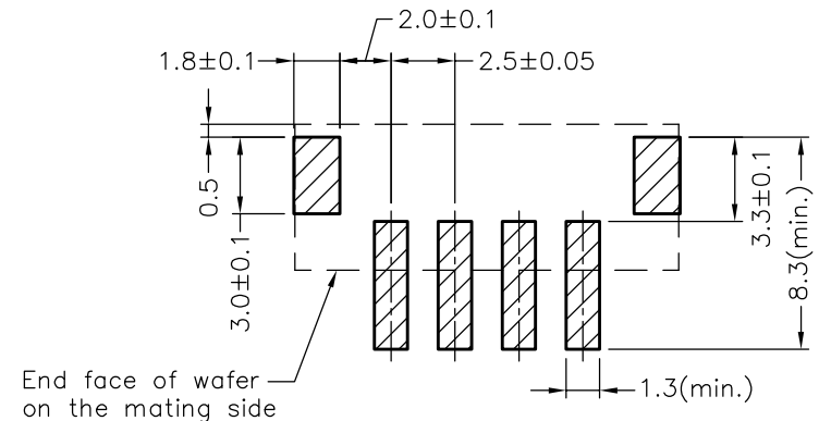
P.C.B LAYOUT
