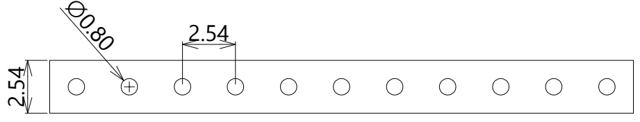
P.C.B LAYOUT
