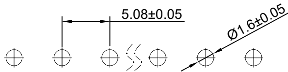
P.C.B Hole Layout
