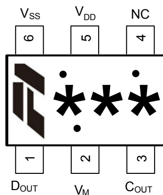
顶视图
