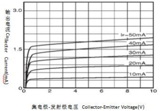
输出特性
