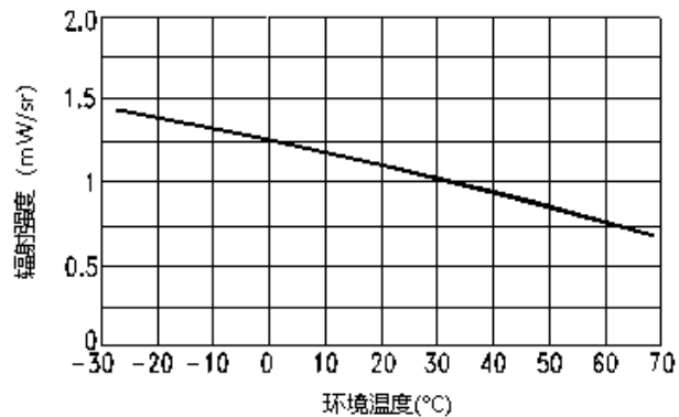
图六：相对辐射度和环境温度关系曲线
