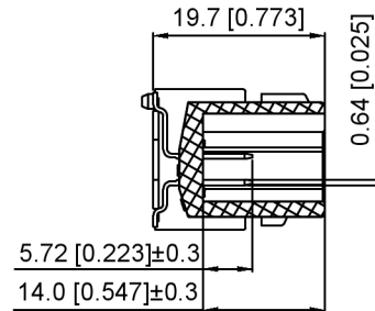
SEC:A-A
