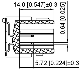
SEC:A-A
