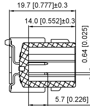
SEC:A-A
