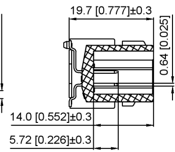
SEC:A-A
