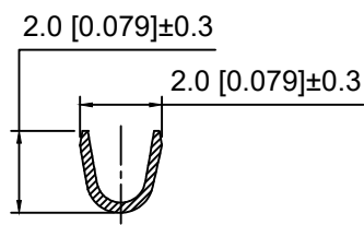
SEC:B-B
