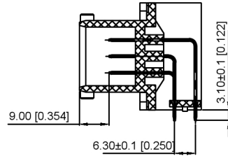
剖面A-A
