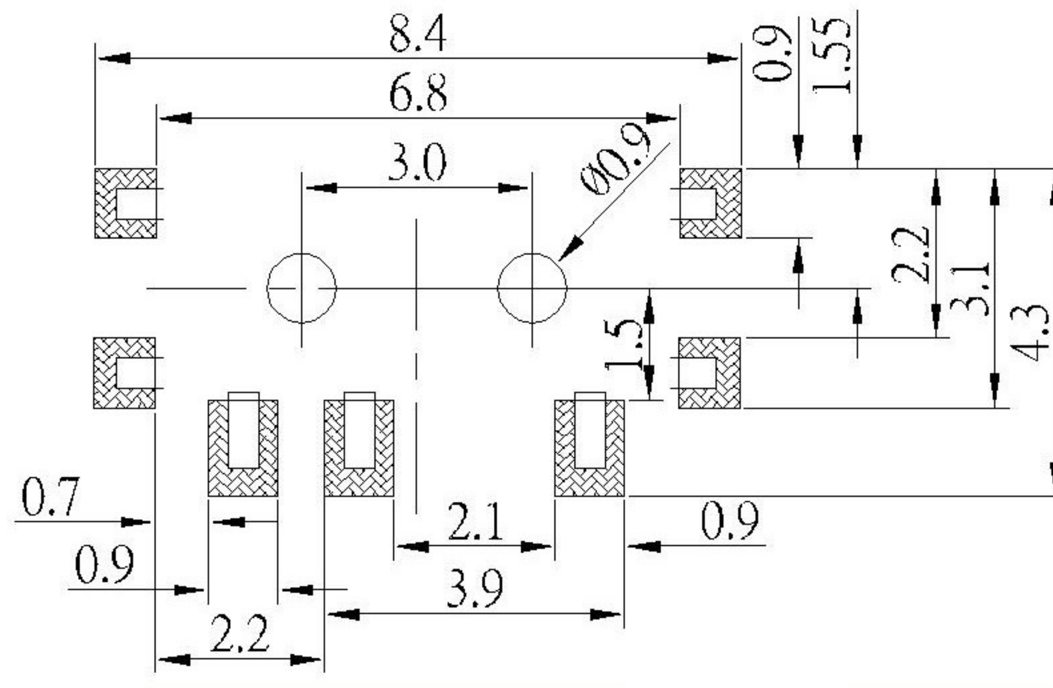
P.C.B LAND PATTERN
