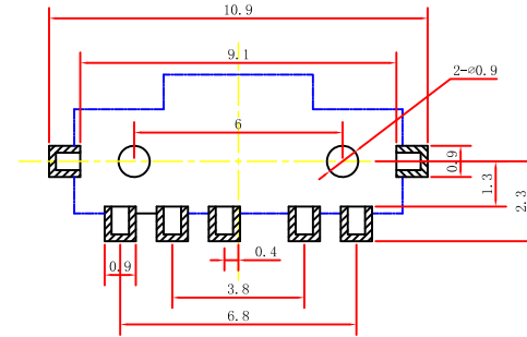
PCB板位置尺寸
