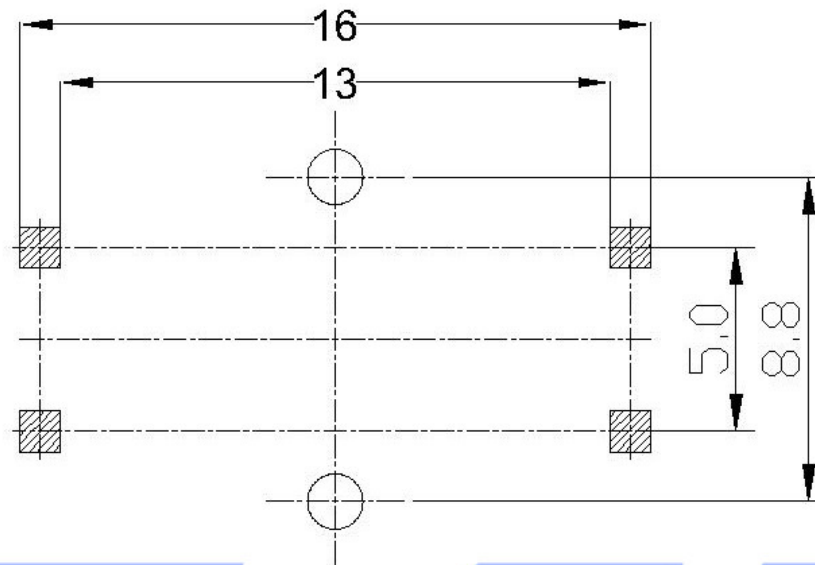
P.C.B. LAYOUT
