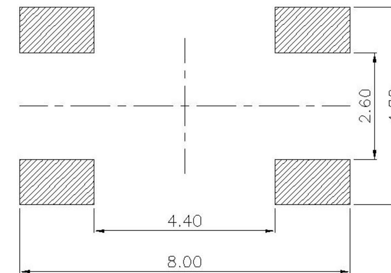
PCB Layout(Pattern side)
