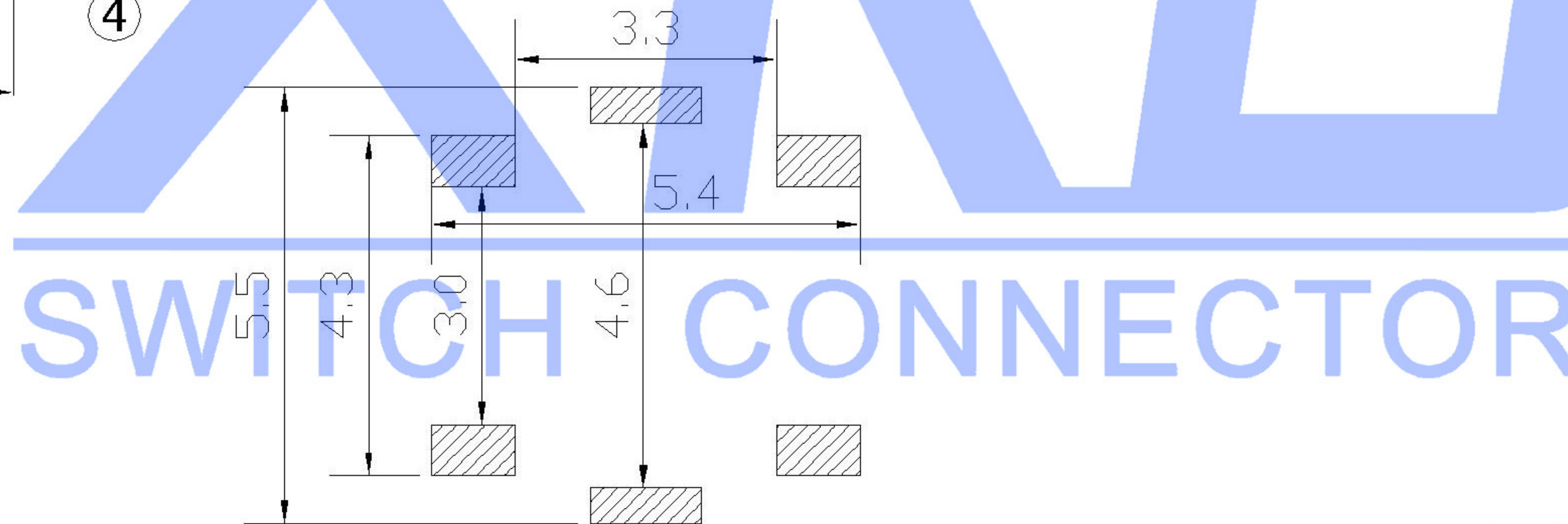
P.C.B. Layout
