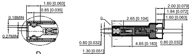
SECT A-A
