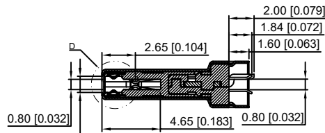
SECT A-A
