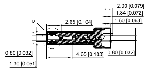
SECT A-A
