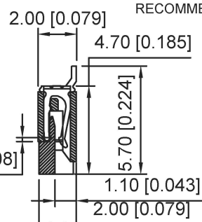
SECTION A-A 下接触
