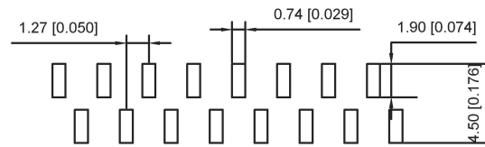
P.C.B LAYOUT(R1)
