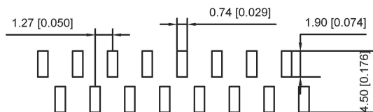
P.C.B LAYOUT(R1)
