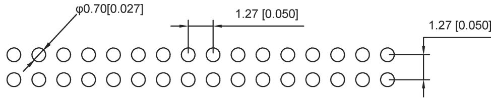
P.C.B LAYOUT
