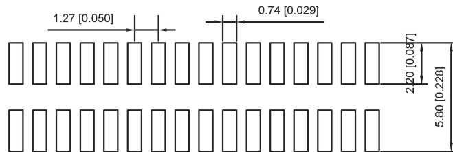
P.C.B LAYOUT
