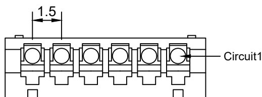
端面 X1502H-XX-N0
