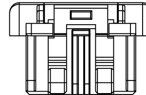
2x06P~2x09P 视图 Scale : 1:1
