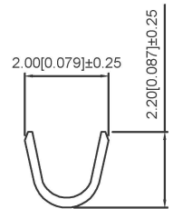
SEC:A-A
