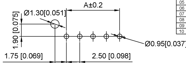
P.C.B LAYOUT
