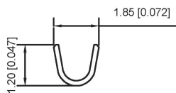
SECTION: B-B SCALE: 1:1
