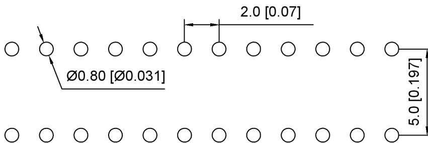
P.C.B LAYOUT
