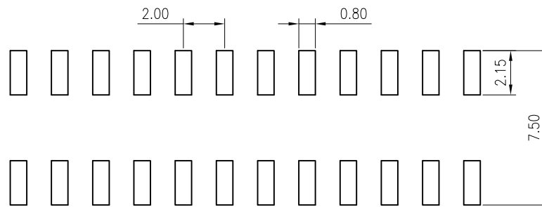
P.C.B LAYOUT
