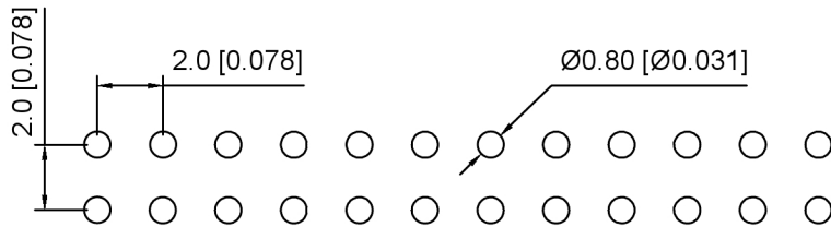
P.C.B LAYOUT
