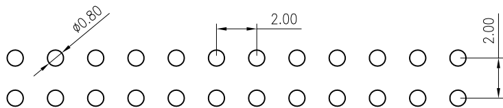
P.C.B LAYOUT
