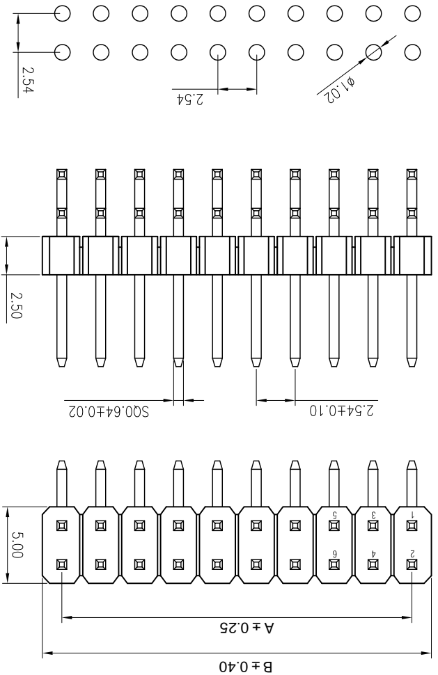
P.C.B LAYOUT
