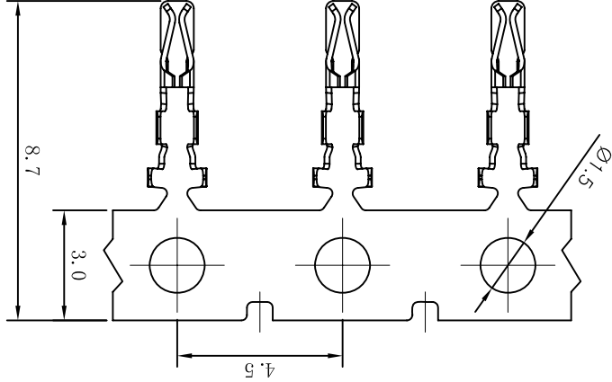
排樣圖 SCALE 0.5:1
