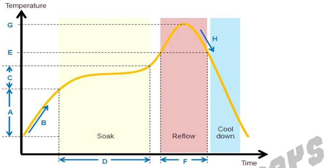
图 10-1 AXP313A 典型回流焊曲线
