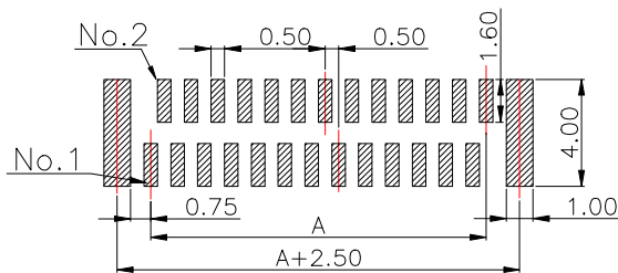
PCB 寸法 (公差±0.05) PCB Layout
