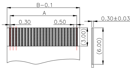
通用FFC寸法 (公差±0.05) Applicable FFC
