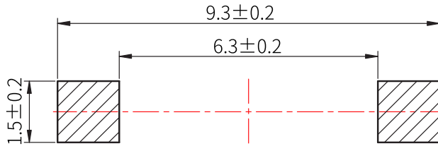
RECOMMENDED P.C.B LAYOUT 安装尺寸图
