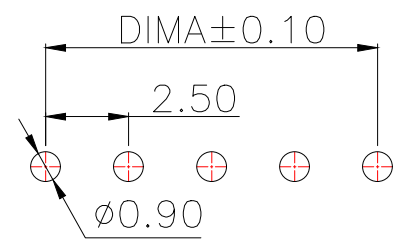
适用线路板(PCB LAYOUT)
