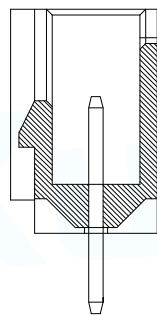
SECTION A-A
