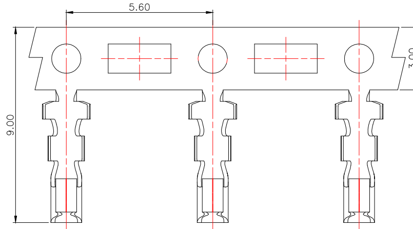
料带图 比例:1:2
