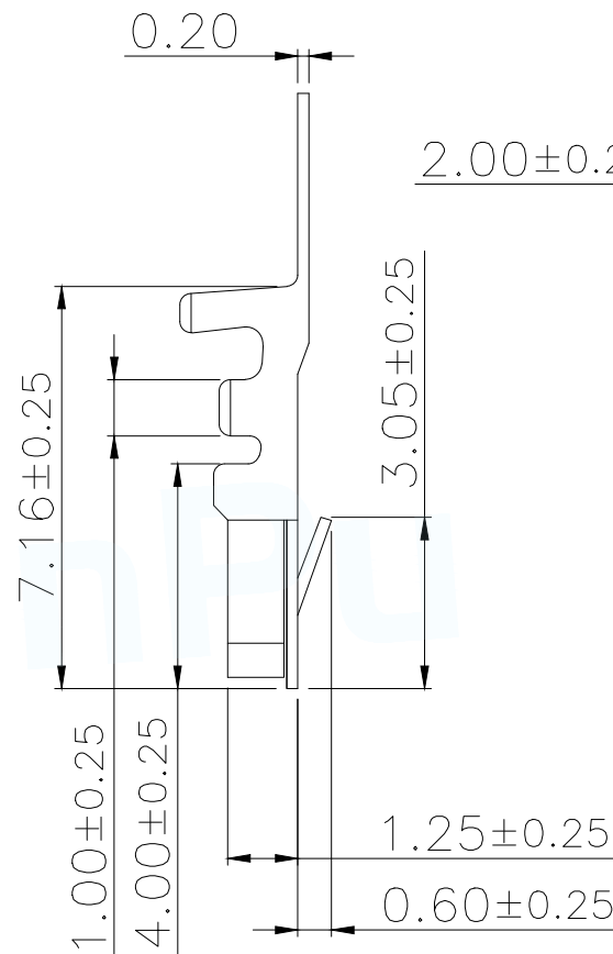
SEC:A-A
