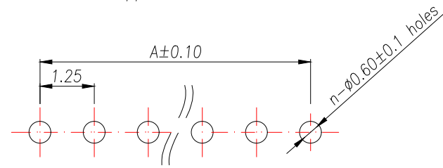
PCB寸法 PCB Layout
