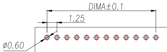
通用线路板(PCB LAYOUT)
