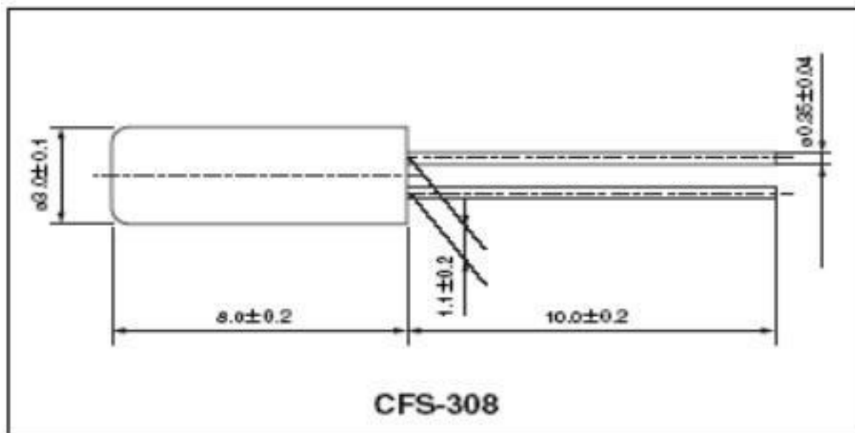
OUTLINE DIMENSIONS(UNIT:mm) 外形尺寸 (单位: mm)
